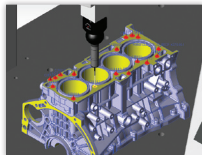
Выбор множества окружностей на одной плоскости осуществляется одним щелчком мыши.
