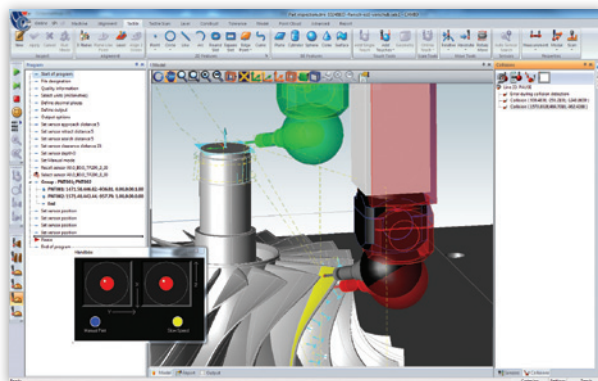
Программы контроля могут быть созданы и апробированы в офлайн режиме.
