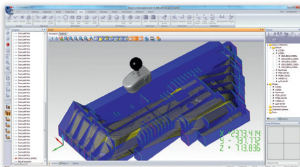
Полное графическое представление траектории планируемого сканирования.
